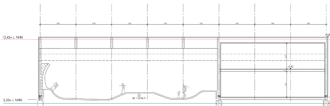
Abbildung 10: Systemschnitt Variante Halle, Blick aus Osten
