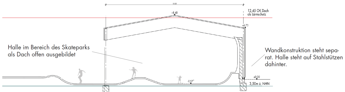
Abbildung 9: Systemschnitt Variante Halle, Blick aus Süden
