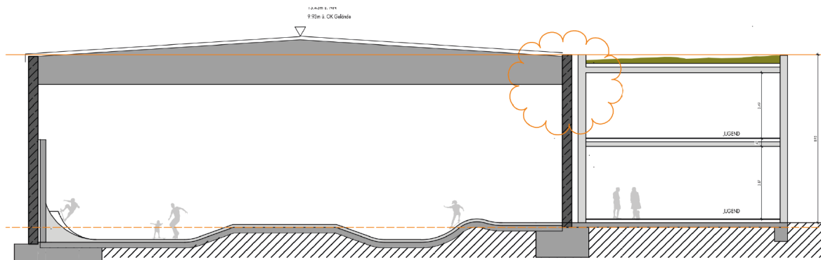
Abbildung 12: Systemschnitt Variante Überdachung, Blick aus Osten
