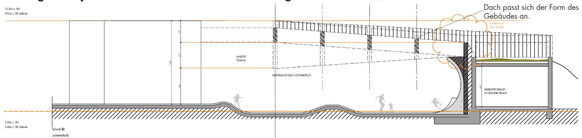
Abbildung 13: Systemschnitt Variante Überdachung und Gebäude, Blick aus Süden
