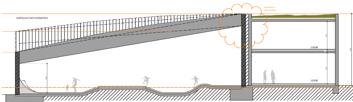
Abbildung 14: Systemschnitt Variante Überdachung und Gebäude, Blick aus Osten
