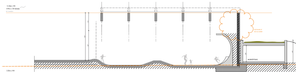
Abbildung 11: Systemschnitt Variante Überdachung, Blick aus Süden
